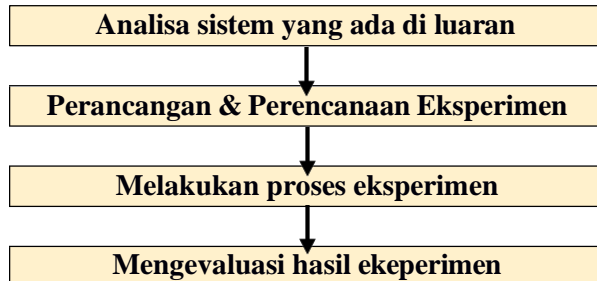
Gambar 3.1. Metodologi Penelitian
