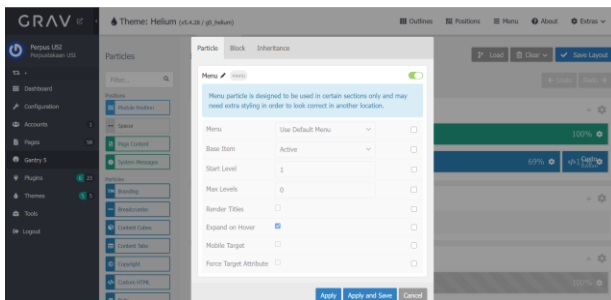
Gambar 2. Pembuatan Header
