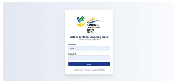
Gambar 7. Halaman Login
